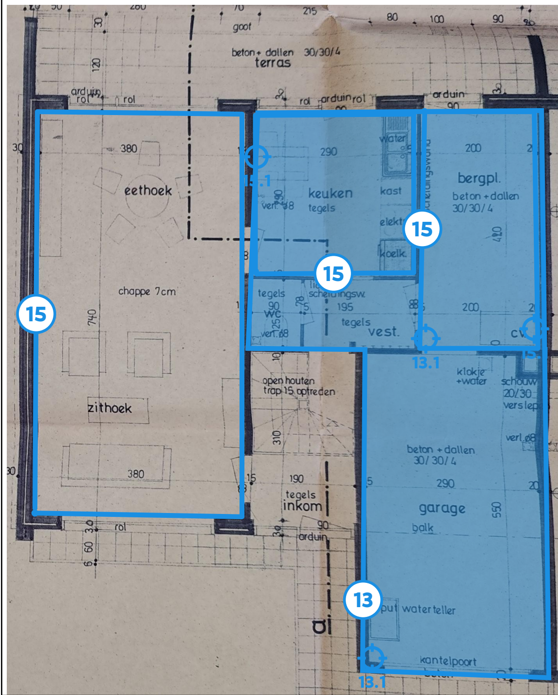
Legende van plan 1.5: A1 - GLV (pleisterwerk muren en plafonds)
